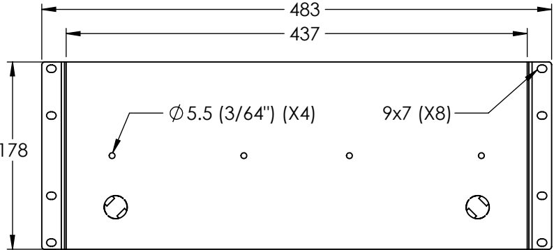
VISTA FRONTAL (SOPORTE)
